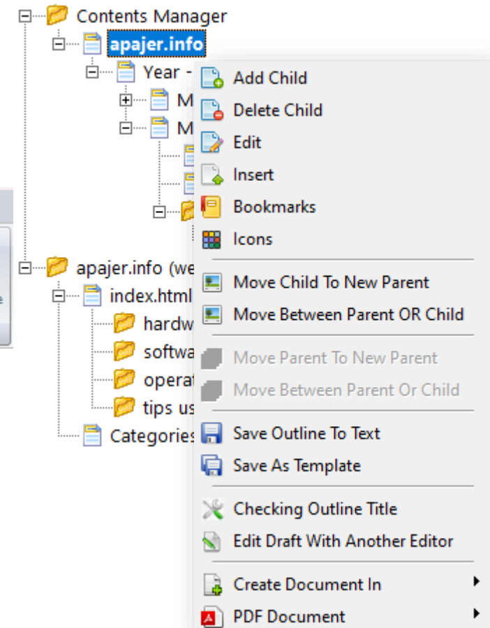
Sub menu
